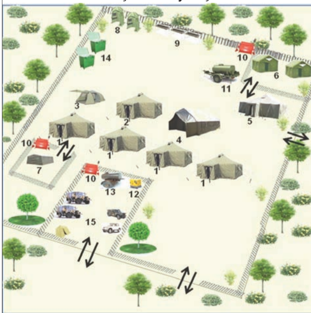
Hərbi hissənin səhra şəraitində yerləşdirilməsinin sxemi
